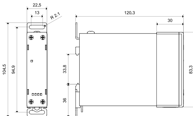
Tipo 77.x5 Morsetti a piastrina
