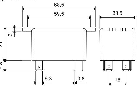
Tipo 66.82-0600
