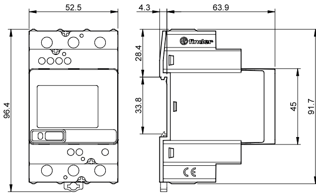
Tipo 7M.38.8.400.0312
