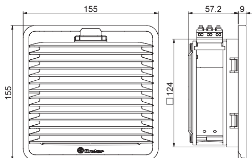
Tipo 7F.20.x.xxx.2055
