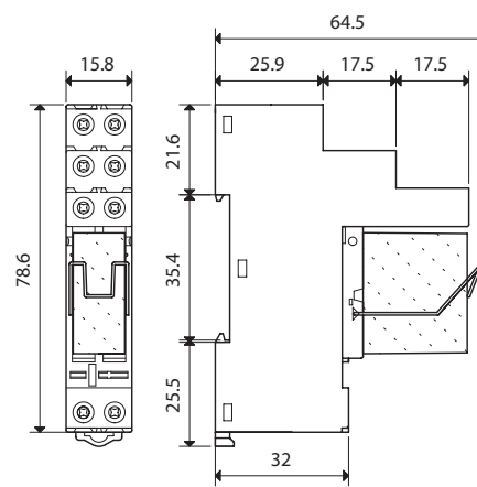
Tipo 48.12 Morsetti a vite
