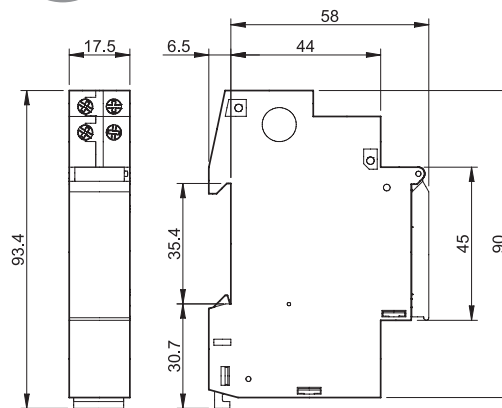
Tipi 12.51/12.81 Morsetti a vite
