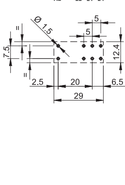
Vista lato rame Lunghezza pin 5.3 mm per zoccolo o montaggio su circuito stampato Vedere codificazione
