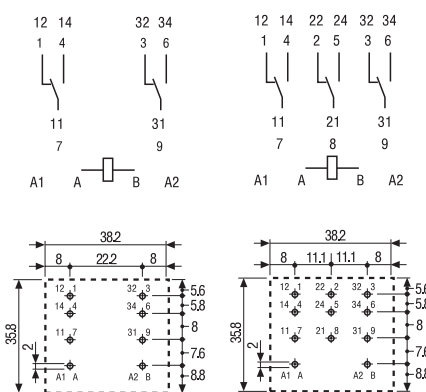
62.22 Vista lato rame 62.23 Vista lato rame
