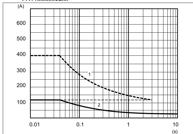
L77-11 Corrente di picco (AC) in funzione della durata 77x5.x.xxx.8x50
