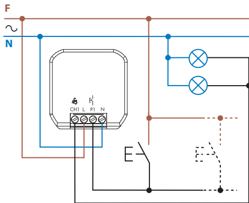
Tipo 15.71 - ollegamento a 4 fili
