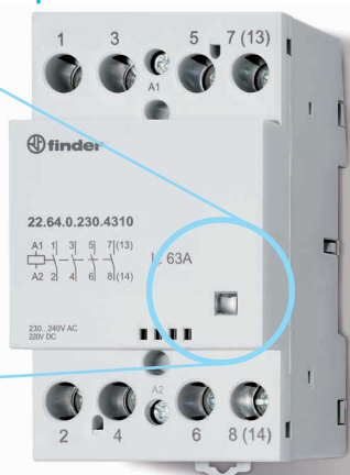
Tipo 22.44 / 22.64 / 22.72 / 22.74
