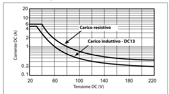
H 7S43* - Massimo potere di rottura su carichi in DC - 7S.43/63
