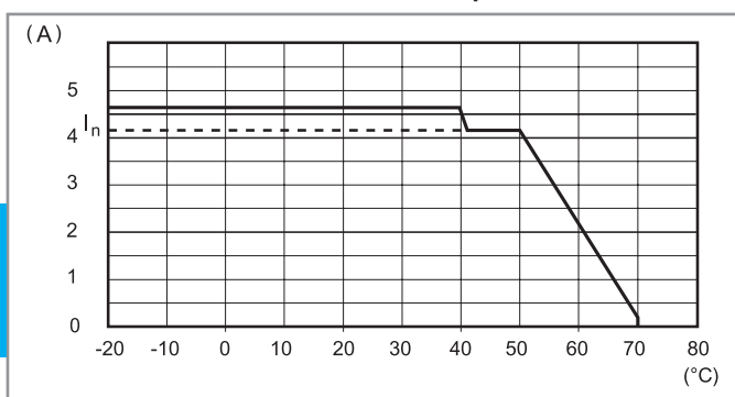
L78-5 Corrente di uscita in funzione della temperatura ambiente (78.50/51)
