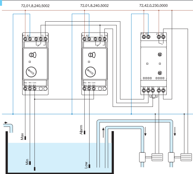
Tipo 72.01/11 Morsetti a vite
