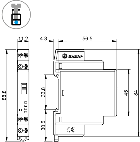
Tipo 19.21 Morsetti a vite
