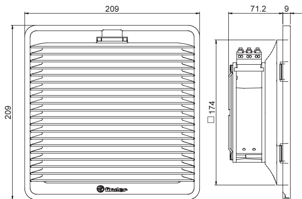
Tipo 7F.20.x.xxx.3100
