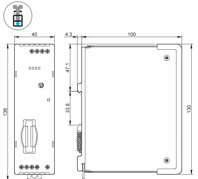
Tipo 78.1B Morsetti a vite
