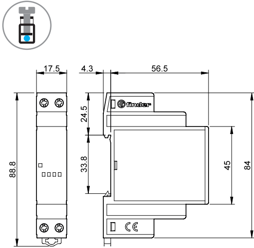
Tipo 78.36 Morsetti a vite
