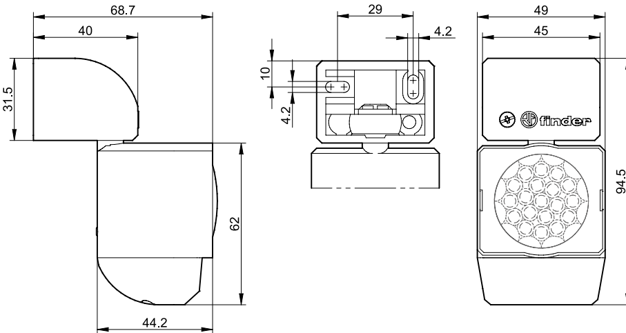
Tipo 18.11
