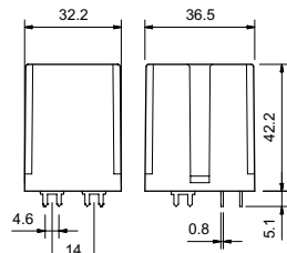
Tipo 65.61
