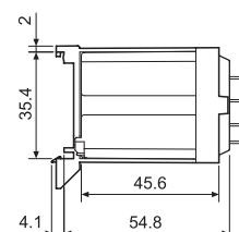
062.07 con relè
