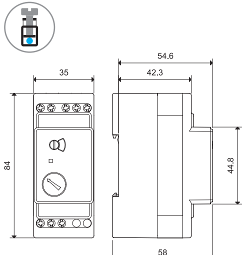
Tipo 72.01/11 Morsetti a vite
