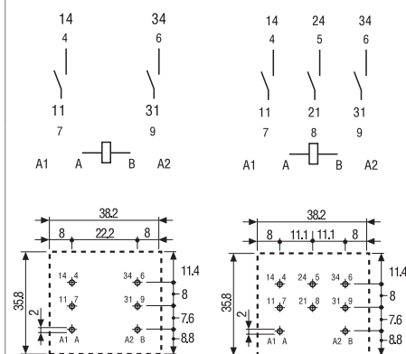
62.22 - 0300 Vista lato rame 62.23 - 0300 Vista lato rame
