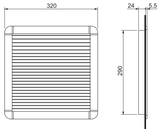
Tipo 7F.05.0.000.5000
