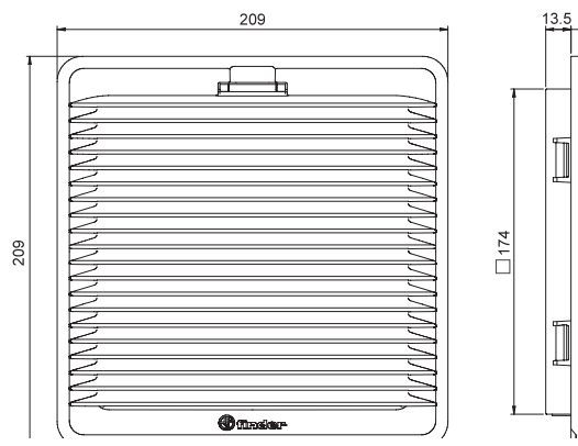
Tipo 7F.02.0.000.3000
