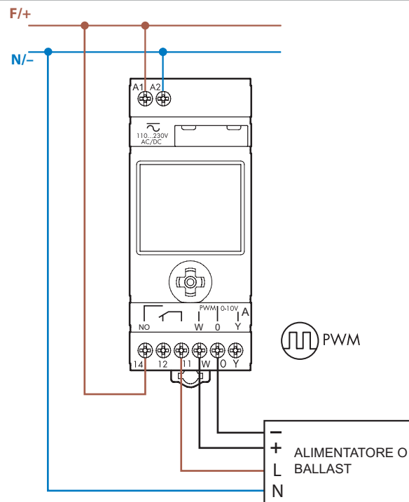
Tipo 12.A4
