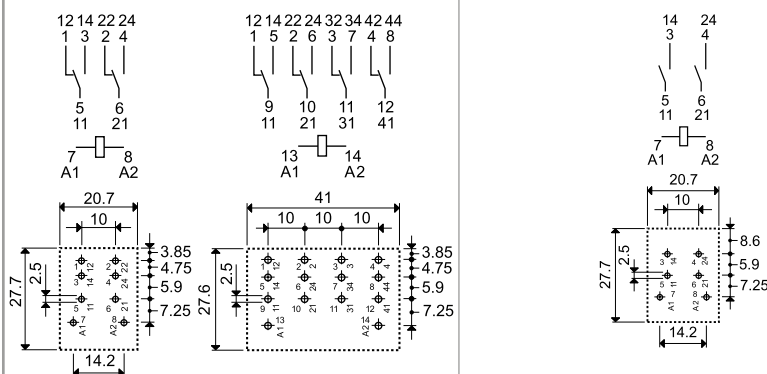
56.42 Vista lato rame
