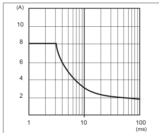
P78-3 Corrente di picco in funzione del tempo (78.36)
