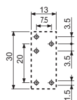
95.13.2 Vista lato rame
