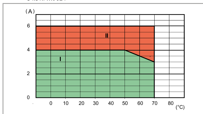
L 34-1 - Corrente DC di uscita in funzione della temperatura ambiente 34.81.7...9024
