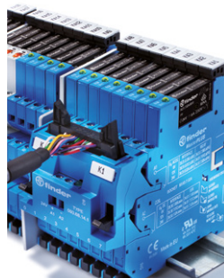
MasterADAPTER connesso
