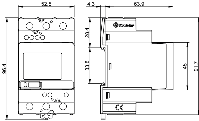
Tipo 7M.38.8.400.0112
