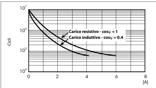
F 39 - Durata elettrica (AC) in funzione della corrente
