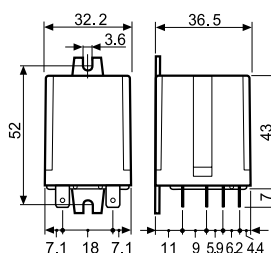
Tipi 60.62
