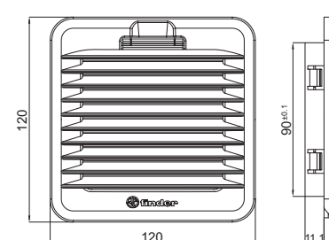
Tipo 7F.02.0.000.1000
