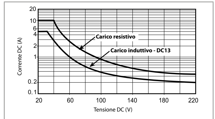
H 7S23* - Massimo potere di rottura su carichi in DC - 7S.23
