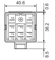
062.07 con relè
