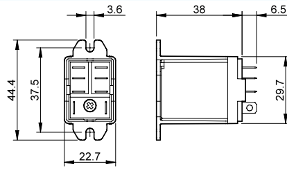
056.25 con relè
