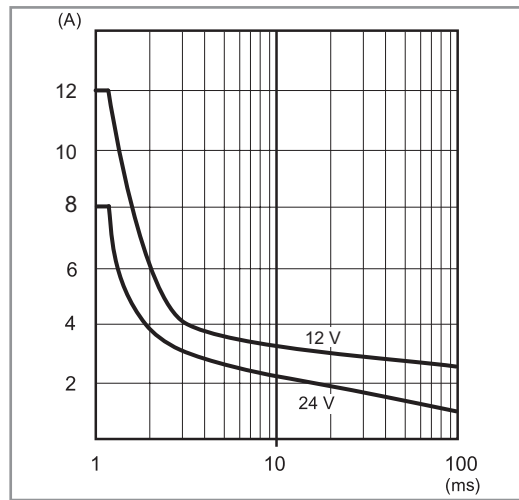
P78-3 Corrente di picco in funzione del tempo (78.36)
