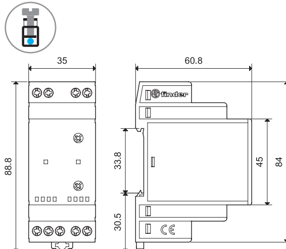
Tipo 72.42 Morsetti a vite
