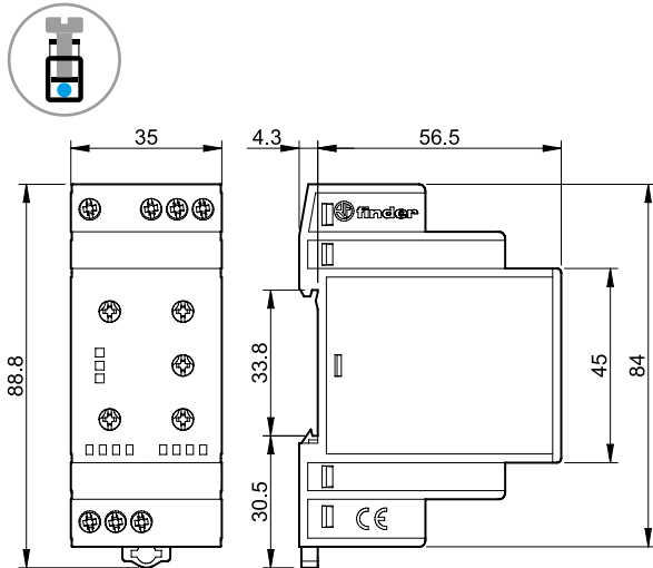
Tipo 70.41 Morsetti a vite
