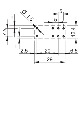
Vista lato rame Lunghezza pin 3.5 mm per circuito stampato Lunghezza pin 5.3 mm per zoccolo o montaggio su circuito stampato Vedere codificazione
