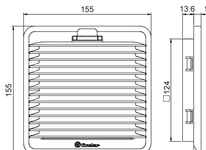
Tipo 7F.02.0.000.2000
