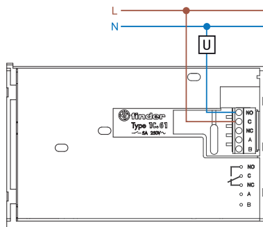
Schema di collegamento
