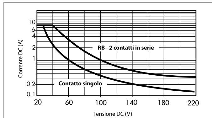
RR - Massimo potere di rottura su carichi in DC1
