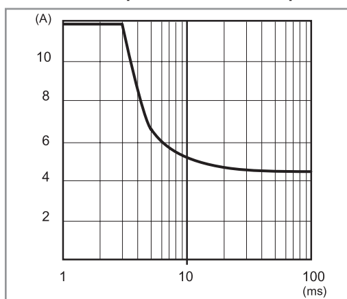
P78-6 Corrente di picco in funzione del tempo (78.61)
