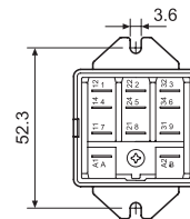
062.05 con relè
