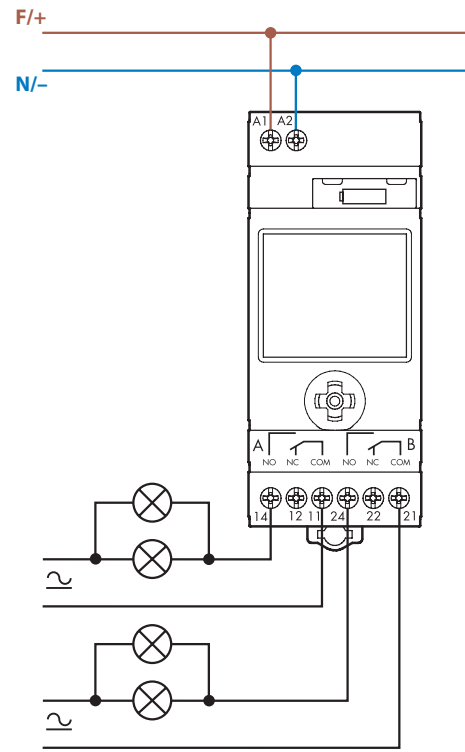
Tipi 12.62 12.A2
