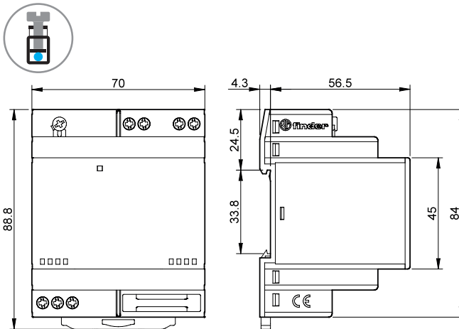
Tipo 78.51 / 78.61 Morsetti a vite
