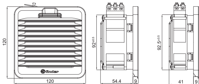
Tipo 7F.20.x.xxx.1020
