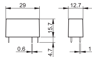
Tipo 41.81-9024/41.81-8240
