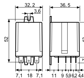
Tipi 60.63
