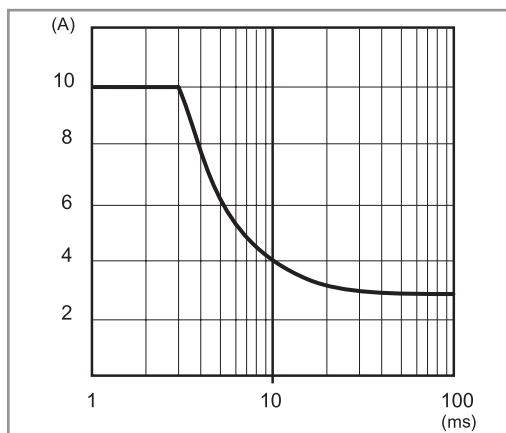
P78-5 Corrente di picco in funzione del tempo (78.50/51)
