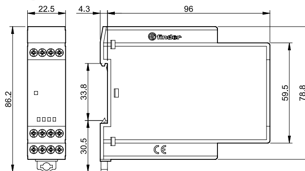
Tipo 75.63 Morsetti a vite
