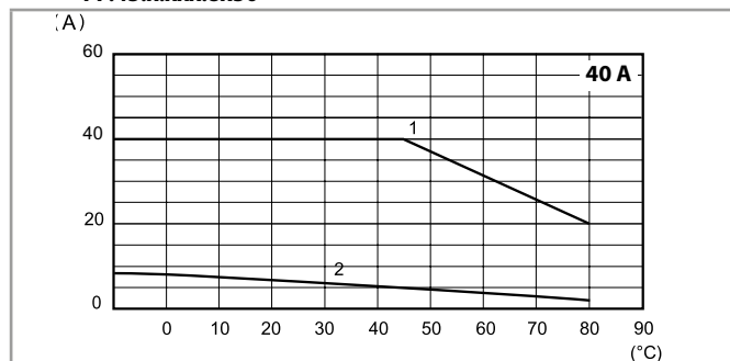
L77-9 Corrente RMS di uscita in funzione della temperatura ambiente 77.45.x.xxx.8x50
