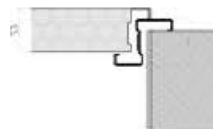
Dettaglio sezione orizzontale
