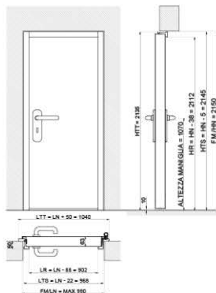
ESEMPIO SISTEMA FORO MURO 990X2140 PORTA METAL EI120
