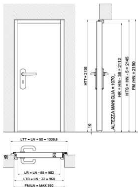
ESEMPIO SISTEMA FORO MURO 990X2140 PORTA METAL USIVARI
