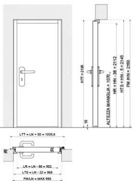
ESEMPIO SISTEMA FORO MURO 990X2140 PORTA METAL EI60
