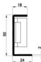
SEZIONE A-A
