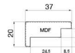
DETTAGLIO TECNICO
